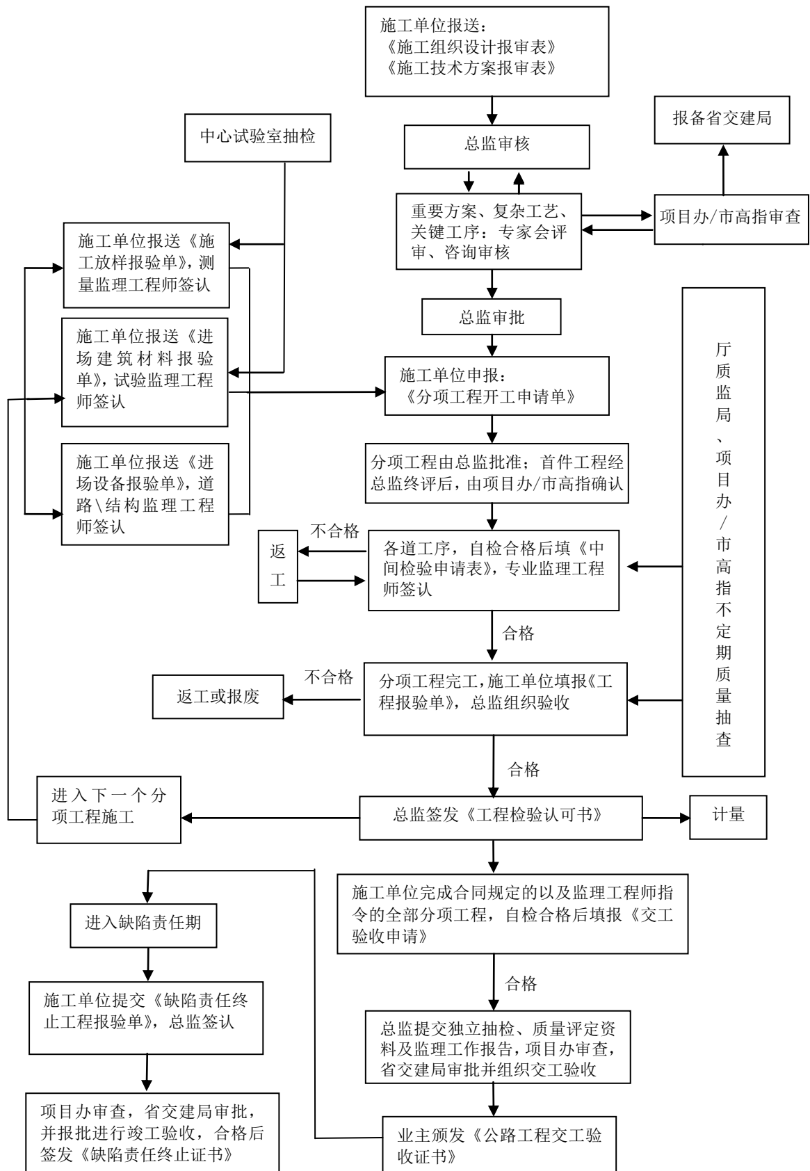
施工质量控制程序流程图
